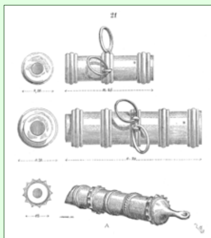
Disegno di cannoni XIV sec. Immagine tratta da wikipedia
